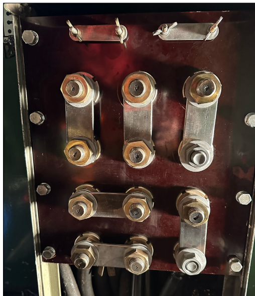
Die neu montierte Klemmplatte in der Lokomotive HGe 4/4 I Nr. 36
